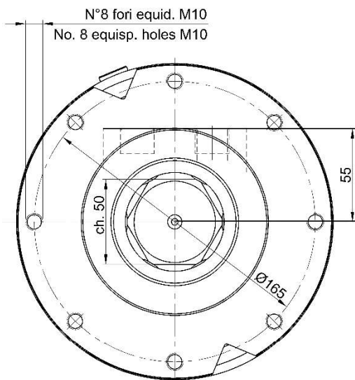
Flangiatura N N flange
